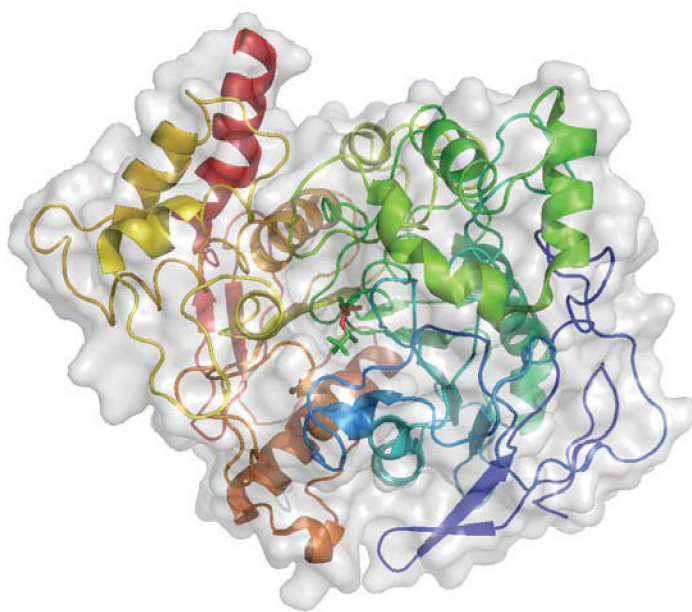
乙酰胆碱酯酶的梭曼接合物。乙酰胆碱酯酶是对神经系统而言至关重要的一种酶。像梭曼这样的神经毒剂可以抑制乙酰胆碱酯酶正常作用。（蛋白质数据库结构2WFZ）
